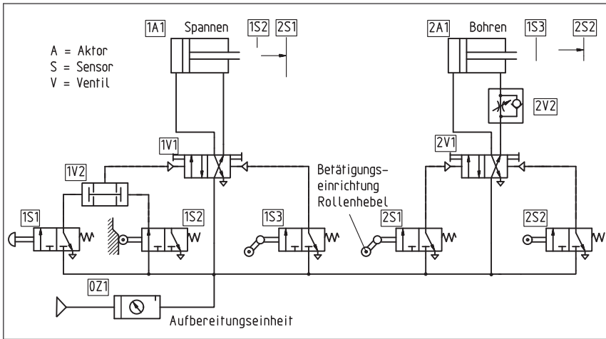
Bild 1.4-2 Schaltplan einer Bohreinrichtung
